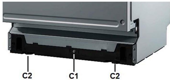
Positionierung Schrauben für Stellfüße 2x Vorne(C2) / 1x Hinten (C1) Positioning screws for levelling feet 2x front (C2) / 1x rear (C1)
