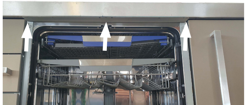
Positionierung Verbindungsschrauben APL 3x Schrauben Positioning connecting screws worktop 3x screws
